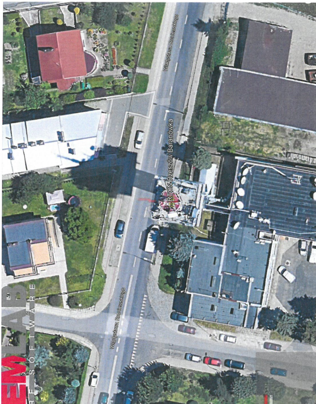
Rys. 2. Rzut poziomy rozkładu pola elektromagnetycznego anteny nowo projektowanej linii radiowej w otoczeniu RTON Rzeszów / Baranówka przewidzianej do zainstalowania na wysokości 42 m nad poziomem terenu.
